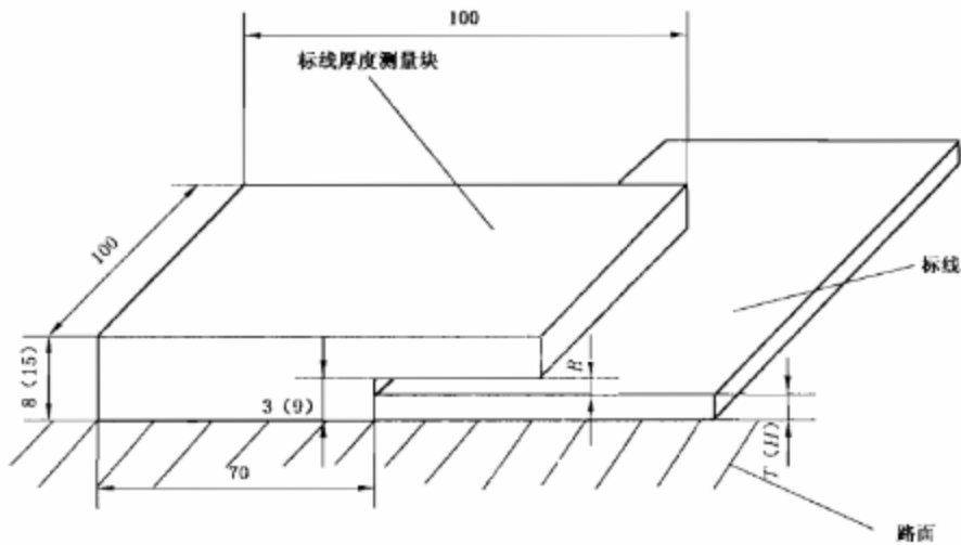
图 A.1 已成形标线厚度测量示意图
