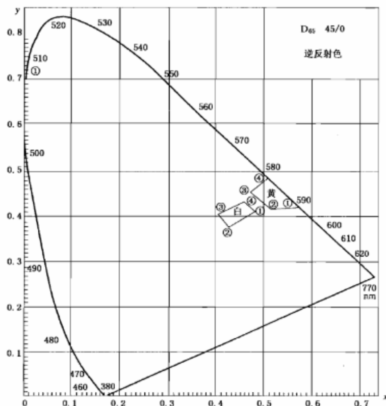
图2 反光标线逆反射色色品图
